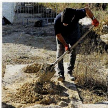
Préparation d'un mortier de chaux et construction d'un muret.
